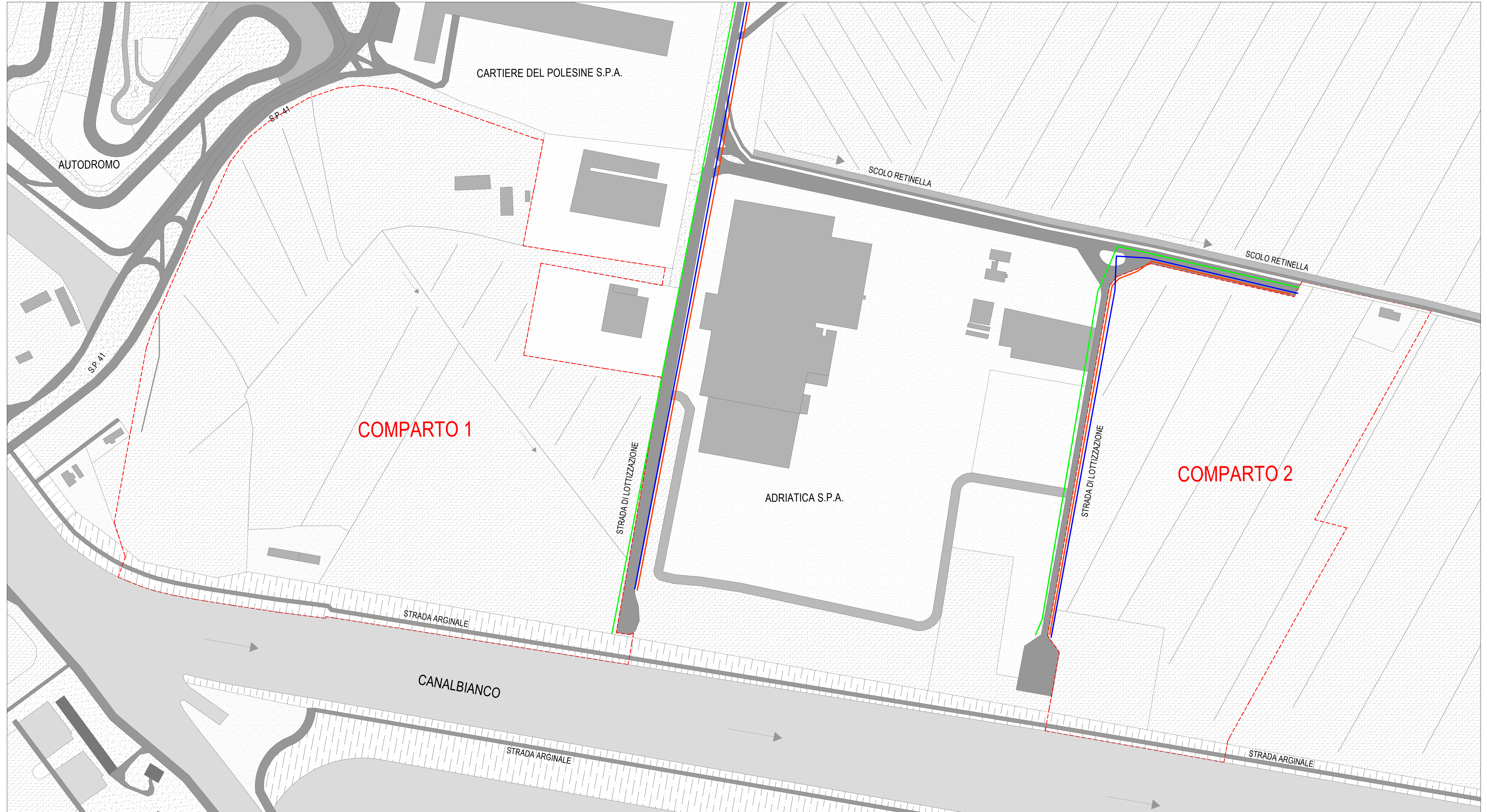
RETI TECNOLOGICHE (acque bianche, acque nere, acquedotto)
